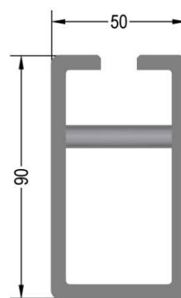
C-Profil 90x50 mm znitovaný
