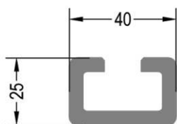
C-Profil 25x40 mm
