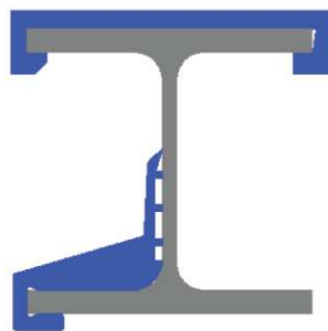
HEB 160
