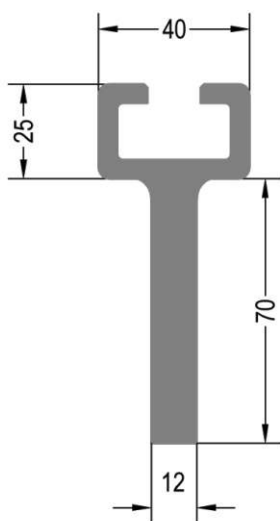
C-Profil 25x40 mm s navarenou plochou oceľou
