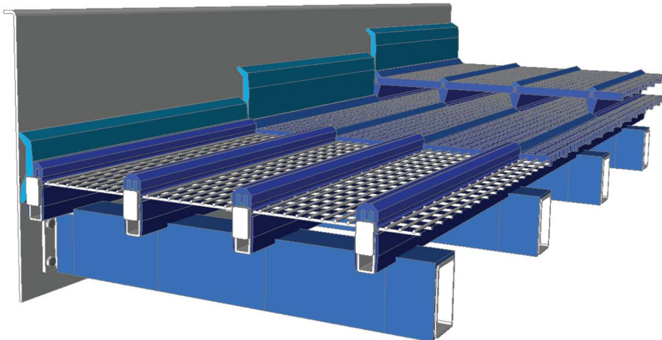
Detail ochrannej plochy
