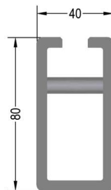
C-Profil 80x40 mm znitovaný
