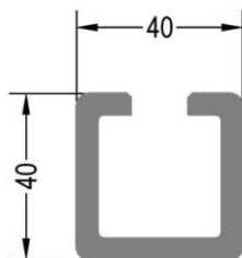
C-Profil 40x40 mm
